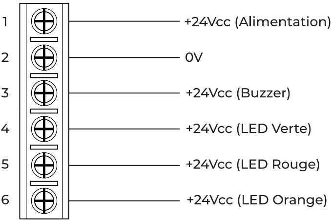
Schéma câblage 1 (Vcc)
