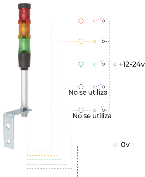
Diagrama eléctrico 2 (BR100)
