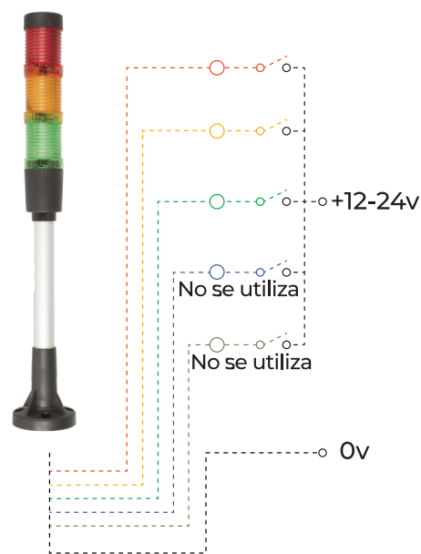
Diagrama eléctrico 1 (FT100)
