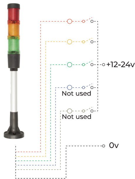
Wiring Diagram 1 (FT100)
