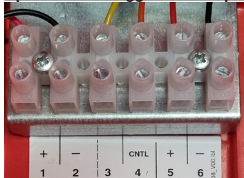
Figura 4: Morsettiera per i collegamenti dell'unità YL
